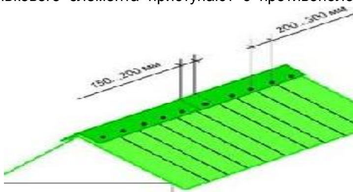
Рис. 10 Крепление конькового элемента
