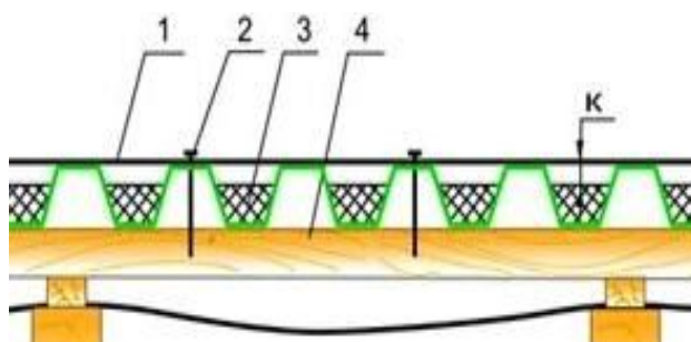
Рис. 11 Конек (продольный разрез)
