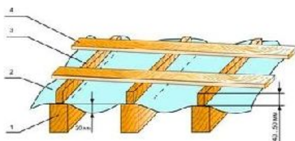
Рис. 4 Укладка гидроизоляции и обрешетки
