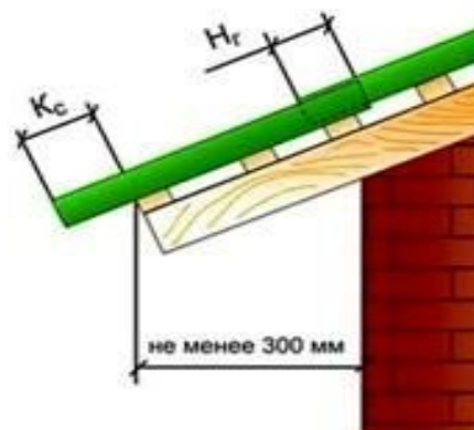
Рис. 1 Карниз кровли
